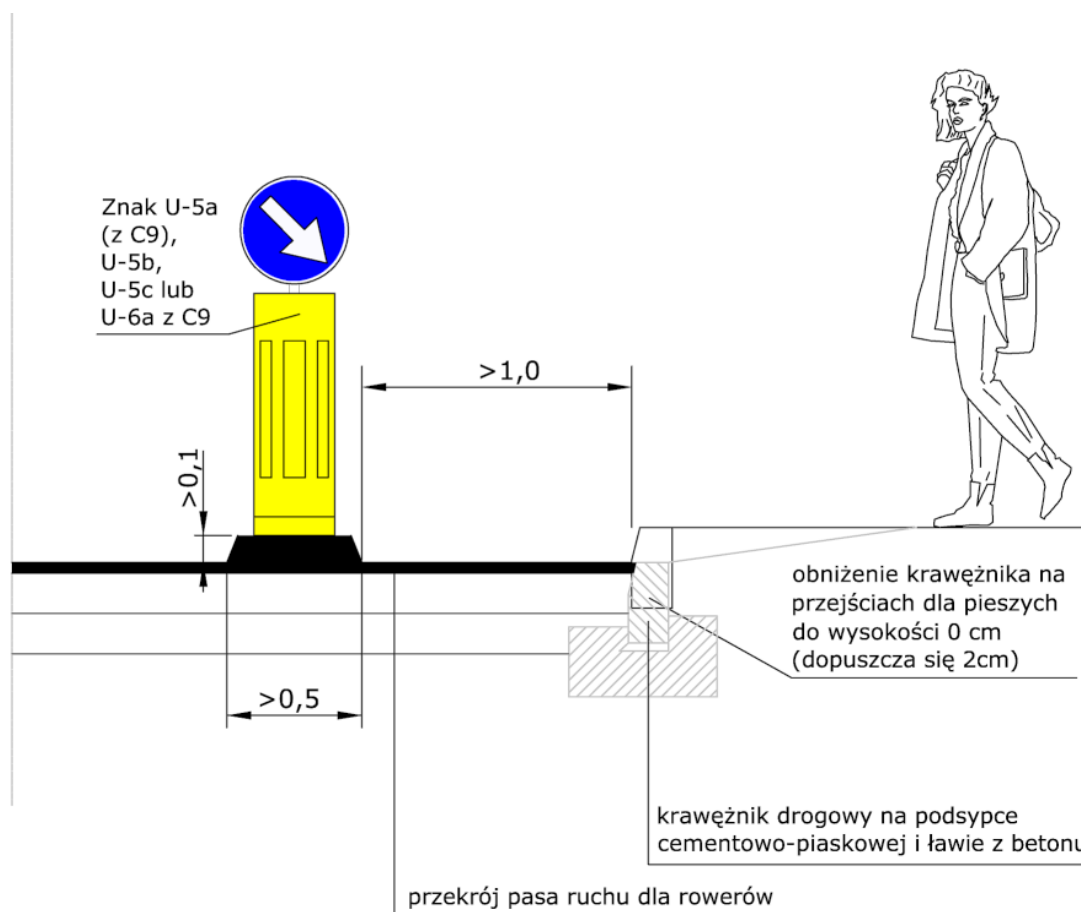
Rys. 11. Wyspa dzieląca ze słupkiem przeszkodowym U-5a/b/c (lub tablicą U-6a) oddzielającą pas ruchu dla rowerów (kontrapas) od pozostałej części jezdni. Widoczne dopuszczalne wyjątkowo zwężenie pasa ruchu dla rowerów do 1,0 m w poziomie niwelety.
