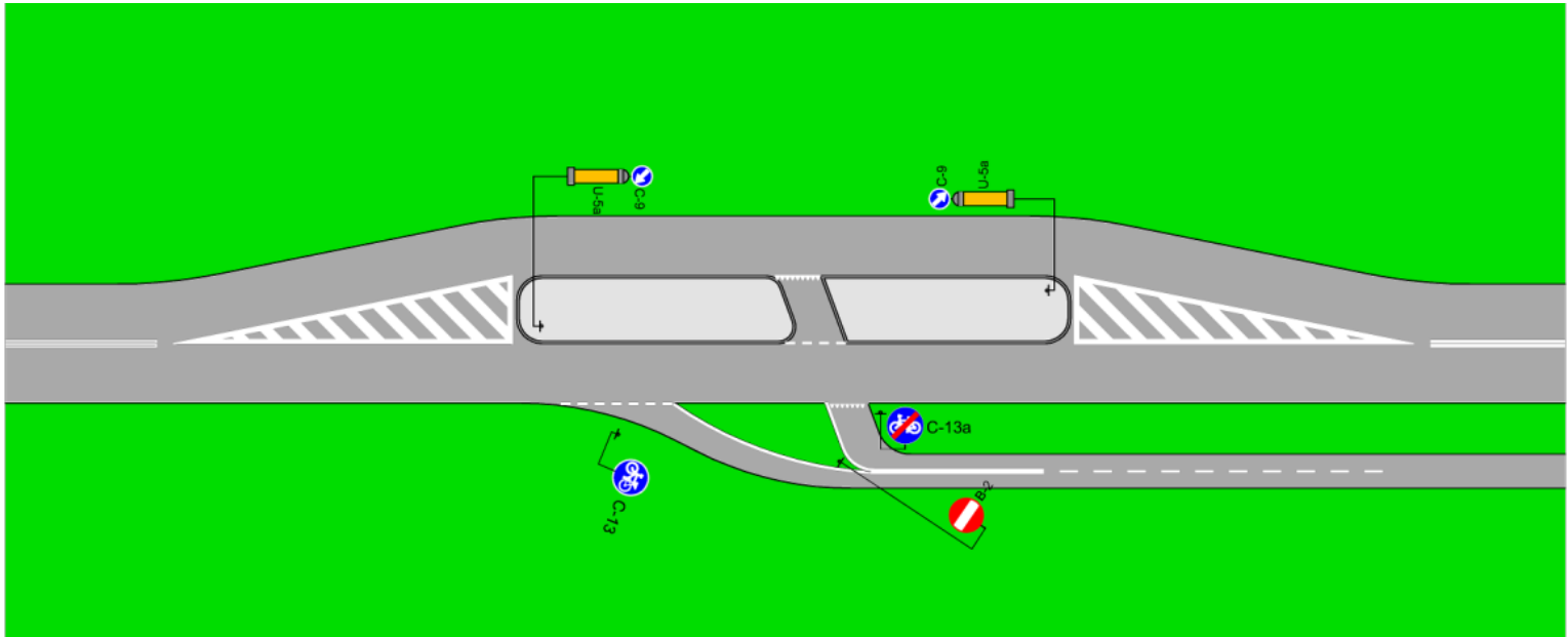
Rys. 17D. Zakończenie dwukierunkowej drogi dla rowerów z wprowadzeniem ruchu rowerów w jezdnię na podporządkowaniu przez azyl wytworzony przez wyspę dzielącą między pasami ruchu. Zjazd z jezdni na drogę dla rowerów odbywa się z zachowaniem parametrów geometrycznych określonych na rysunkach 17A i 17B.
