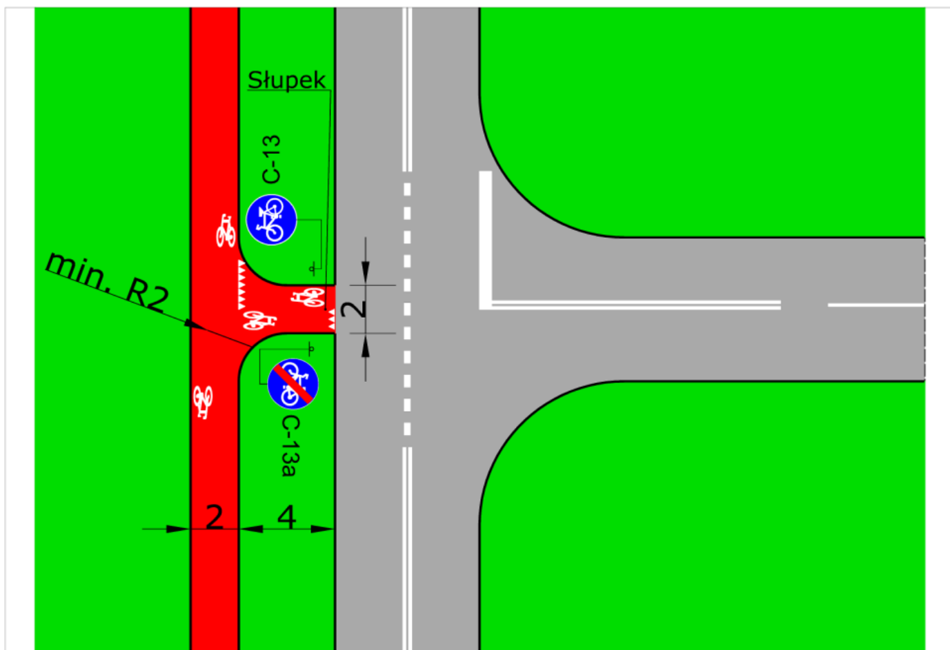
Rys. 23. Przykład drogi z drogą dla rowerów skomunikowaną na skrzyżowaniu w kształcie litery T („teowym”) przez czwarty wlot. Analogiczne rozwiązania należy stosować w przypadku wszelkich innych źródeł i celów podróży zlokalizowanych po stronie przeciwnej niż biegnie droga dla rowerów. (Część oznakowania pominięto).
