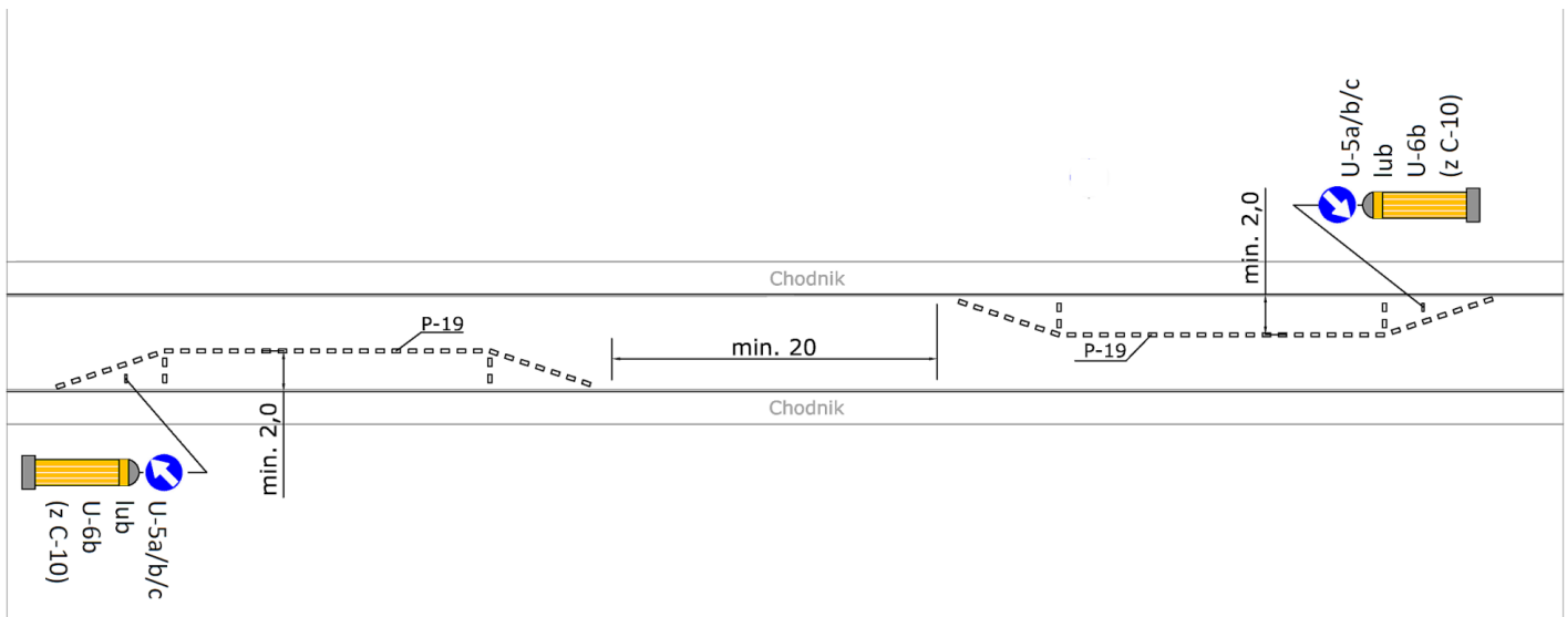
Rys. 3. Esowanie toru jazdy pojazdów przez naprzemienną lokalizację miejsc postojowych.
