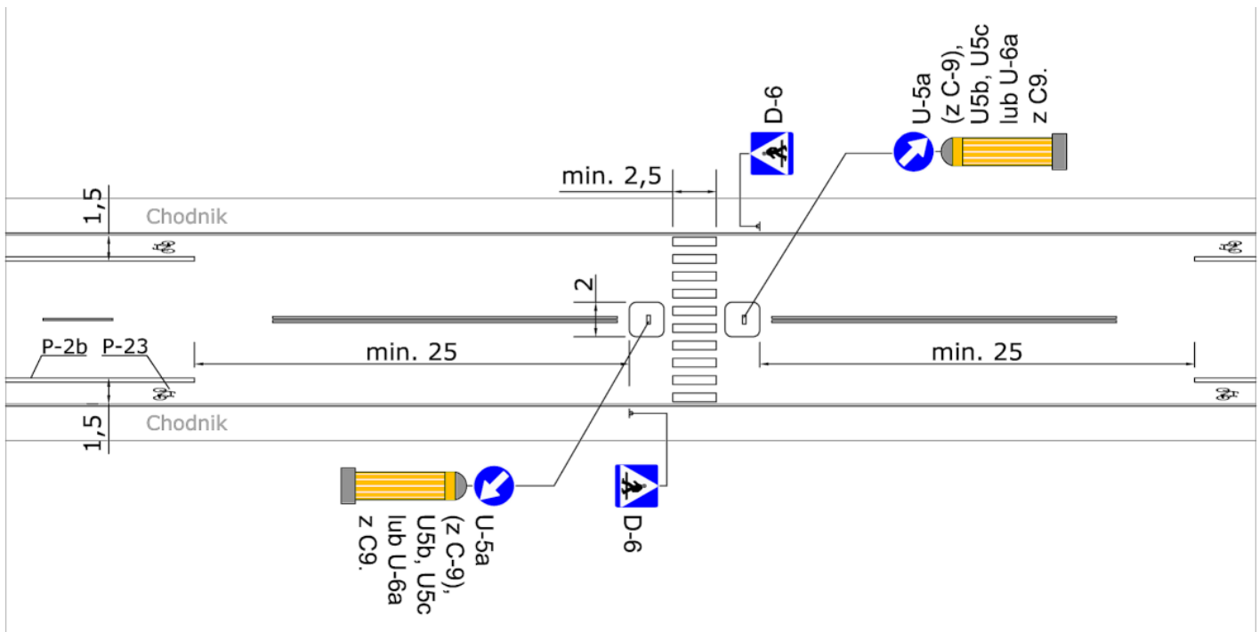
Rys. 9. Przykład prowadzenia pasów ruchu dla rowerów w rejonie przejścia dla pieszych z azylem pośrodku jezdni. Pasy należy zakończyć na 15-20 m przed azylem.
