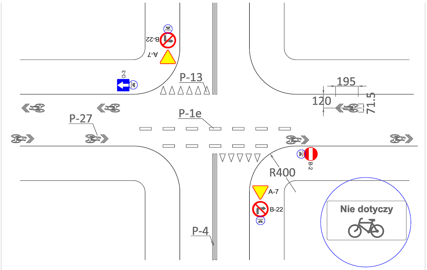
Rys. 4. Przykładowa organizacja dwukierunkowego ruchu rowerowego w jezdni jednokierunkowej – skrzyżowanie z ustalonym pierwszeństwem. Ruch „pod prąd” dopuszczony jest oznakowaniem poziomym P-27, znaki dla kierunku pod prąd umieszcza się zgodnie z opisem w tekście (punkt 4.3), wymiarowanie położenia dla kierunku zgodnego z ogólną organizacją ruchu przedstawiono na rysunku.
