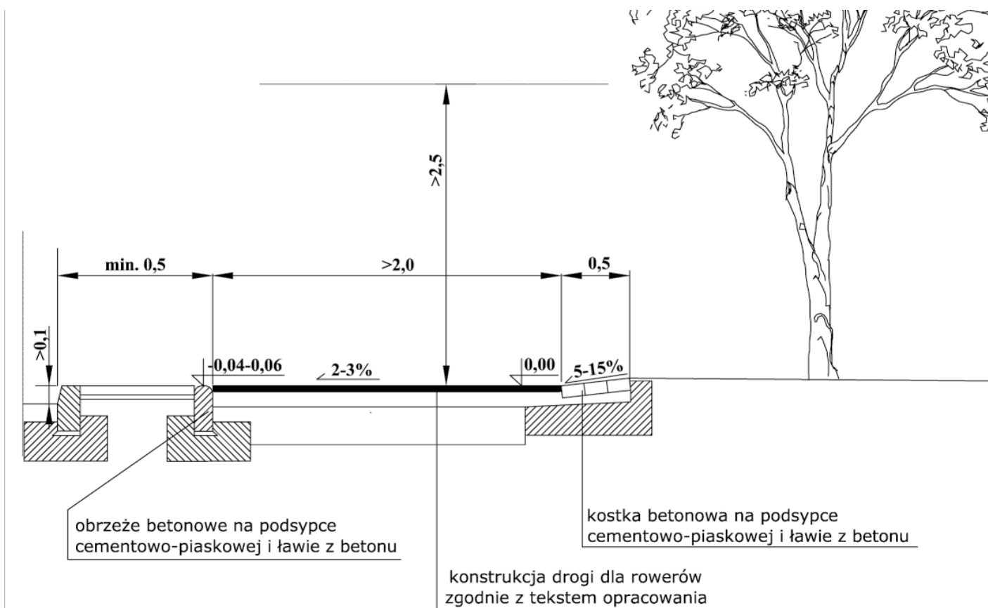
Rys. 12A. Przekrój poprzeczny dwukierunkowej drogi dla rowerów o nawierzchni bitumicznej, zamkniętej obrzeżem i opaską z kostki brukowej oddzielającą ją od chodnika.
