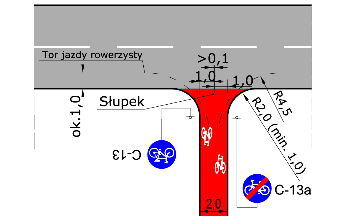
Rys. 17E. Włot dwukierunkowej drogi dla rowerów biegnącej prostopadłe do jezdni ogólnodostępnej z dopuszczonym ruchem rowerów. Aby ułatwić wjazd na drogę dla rowerów i opuszczenie jej zastosowano wyokrąglenia styku krawędzi jezdni ogólnodostępnej i drogi dla rowerów. Na rysunku przedstawiono orientacyjny tor jazdy rowerzystów i położenie słupków blokujących U-12c.
