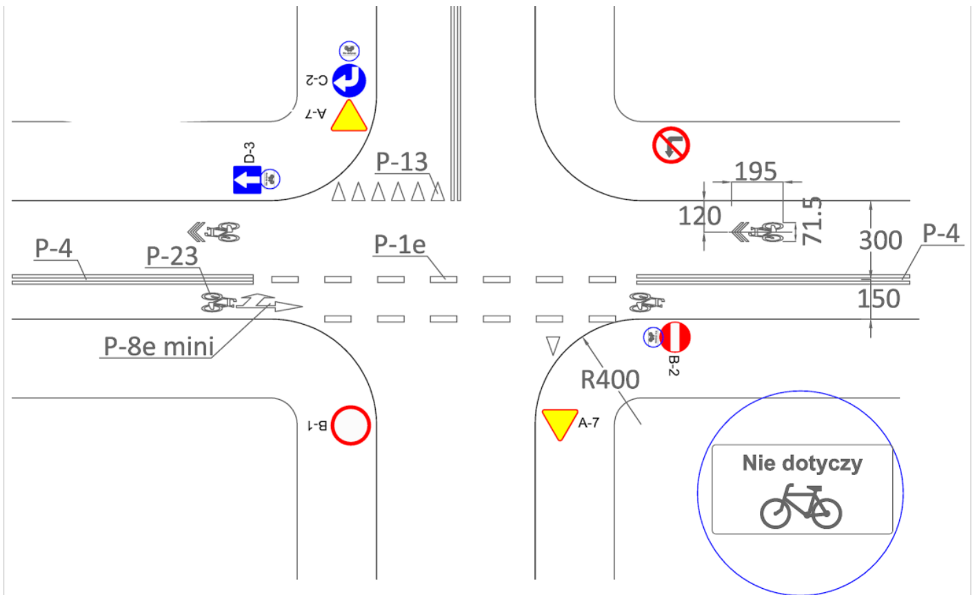
Rys. 10A. Jeśli jazda z kontrapasa jest dozwolona tylko w określonym kierunku, wówczas łącznie ze znakiem P-23 „rower” na wlocie stosuje się odpowiedni wariant strzałki kierunkowej P-8 w rozmiarze mini.
