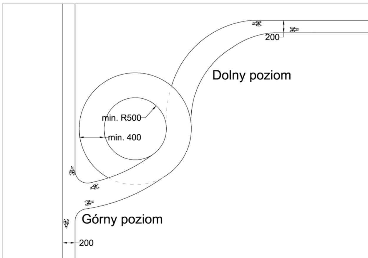
Rys. 24A. Pochylnia ślimakowa łącząca drogę dla rowerów na obiekcie (most, wiadukt, kładka) z niżej położonym terenem. Pochylnia ślimakowa zawsze musi mieć bieg w lewo w dół, co minimalizuje kolizje i poprawia ergonomię. Podany minimalny promień łuku dotyczy ślimaka o planie innym niż kołowy (eliptyczny, nieregularny itp.). W przypadku planu kołowego należy zapewnić aby skok spirali tworzącej ślimak łącznie z przekrojem konstrukcji pochylni uwzględnił skrajnię pionową drogi dla rowerów (2,5 m) a pochylenie podłużne drogi dla rowerów na niej nie przekraczało 5%.
