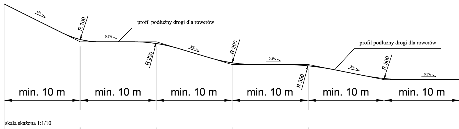
Rys. 15. Przykładowy przekrój podłużny drogi dla rowerów na spadku
