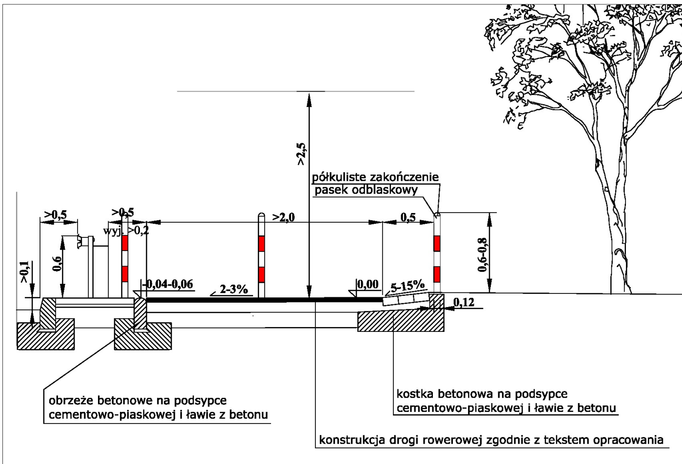
Rys. 13. Zasady lokalizacji słupków blokujących U-12c w przekroju dwukierunkowej drogi dla rowerów. Jeden słupek musi znajdować się symetrycznie w osi drogi dla rowerów. Od jezdni dodatkowo drogę dla rowerów może oddzielać bariera ochronna U-14a.
