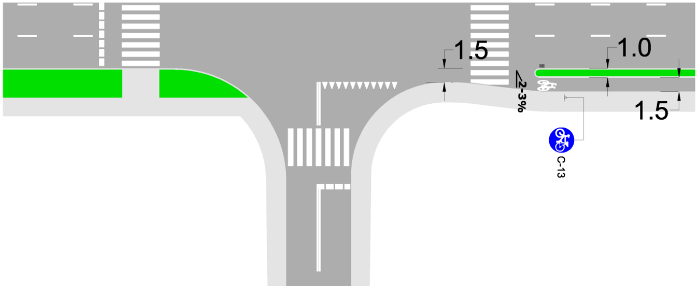
Rys. 17A. Początek jednokierunkowej drogi dla rowerów za skrzyżowaniem z poszerzeniem jezdni
