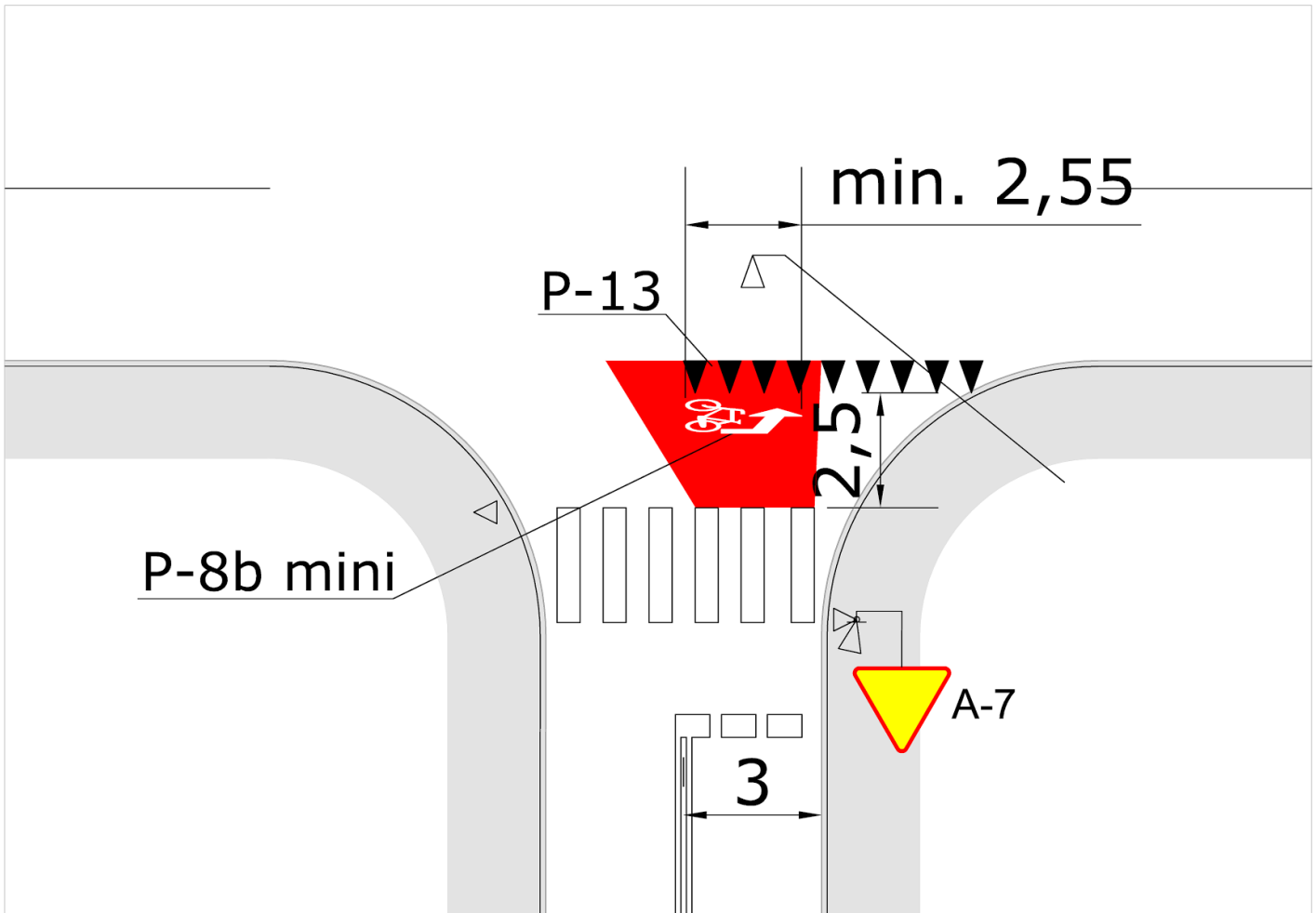
Rys. 20B: Śluza typu 2 zlokalizowana na wlocie podporządkowanym, wloty z pierwszeństwem bez pasa ruchu dla rowerów, przejście dla pieszych przez wlot podporządkowany i sygnalizacja świetlna. Czerwona nawierzchnia śluzy nie jest zwymiarowana (nie stanowi znaku drogowego).
