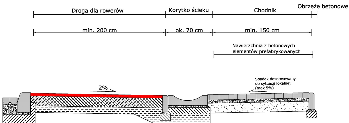
Rys. 12D. Przykład konstrukcji drogi dla rowerów oddzielonej od chodnika prefabrykowanym otwartym ściekiem korytkowym o przekroju wycinka koła.
