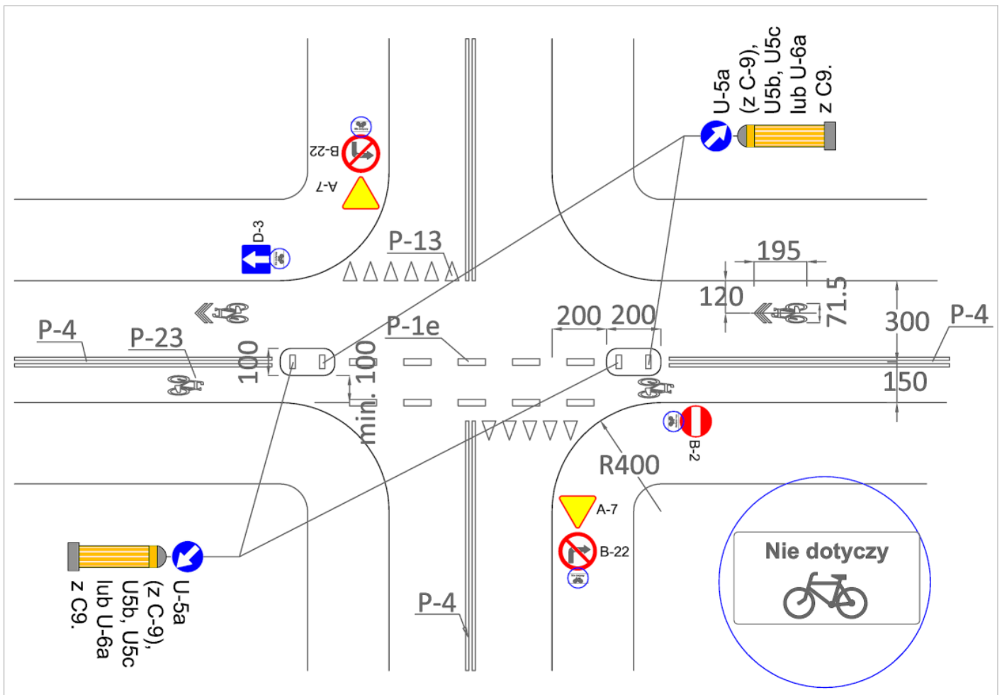
Rys. 10B. Przykład kontrapasa z wyspami dzielącymi na wlotach (porównaj z rys. 11).
