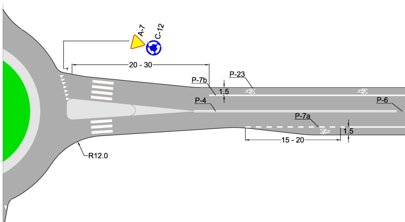
Rys. 18A. Małe rondo z wlotem na którym pas ruchu dla rowerów został obcięty.
