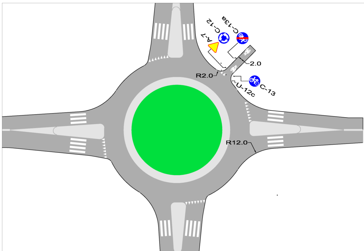
Rys. 18B. Dwukierunkowa droga dla rowerów jako samodzielny wlot małego ronda.
