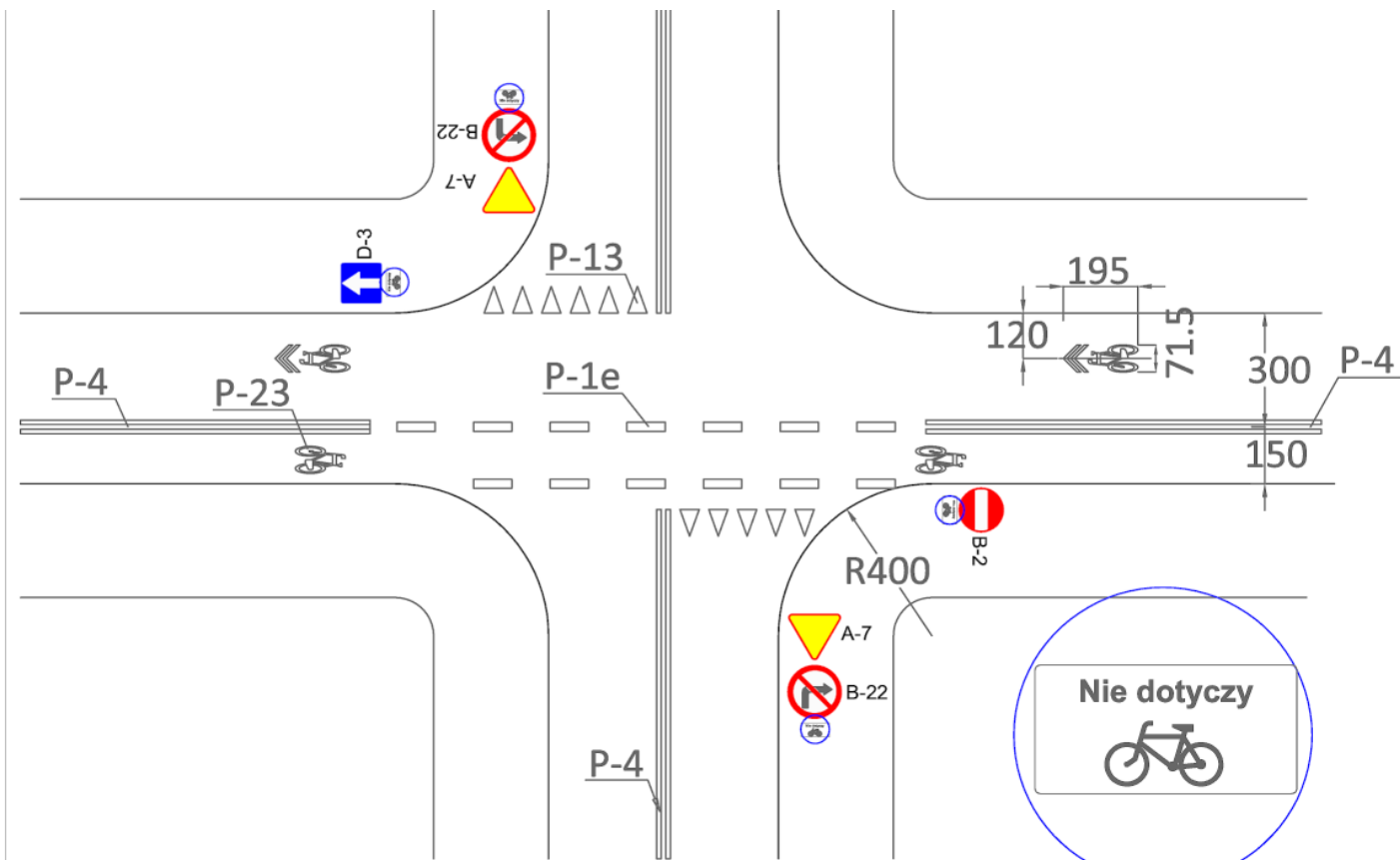
Rys. 10. Kontrapas wyznaczony w jezdni ulicy jednokierunkowej na skrzyżowaniu z ustalonym pierwszeństwem. Jeśli na skrzyżowaniu występuje duże natężenie pojazdów samochodowych na relacji skrętnej z drogi z pierwszeństwem, na wlocie umieszcza się wyspę dzielącą ze słupkiem U-5a/b/c (patrz rys. 10B).
